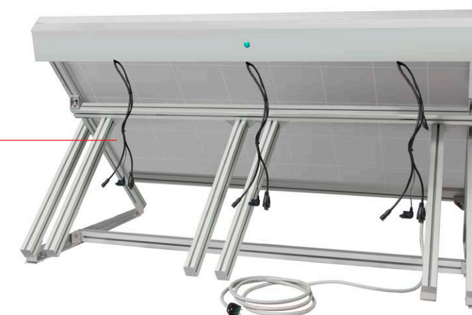
TYP2. MIT STROMNETZ VERBUNDEN IM PLUG & PLAY MODUS
